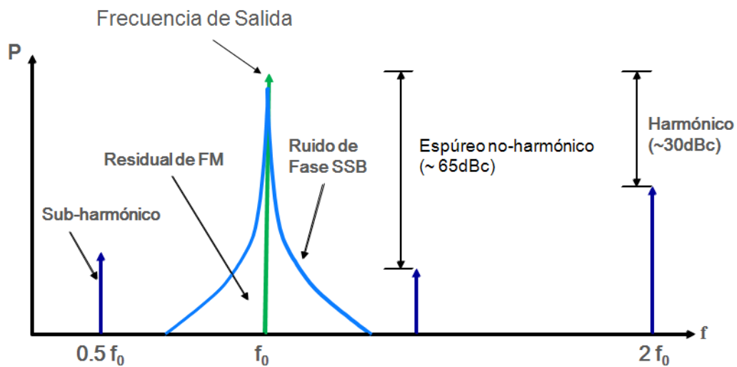
Figura 8. Frecuencia de salida y componentes de la pureza espectral de un generador de señal.
