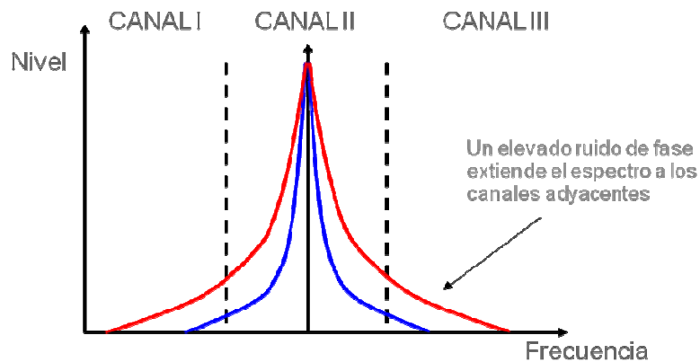
Figura 9. El ruido de fase SSB puede afectar a los canales adyacentes
