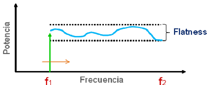
Figura 5. El Flatness se define como la variación del nivel de salida con la frecuencia con respecto a un nivel, normalmente, de baja frecuencia.
