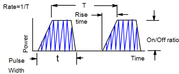
Figura 11. Modulación por Pulsos.
