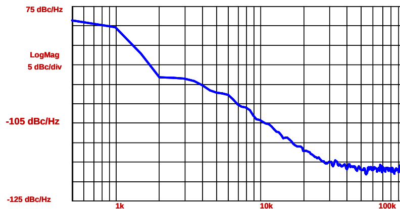
Figura 7. El ruido de fase SSB con respecto a la distancia a la portadora.
