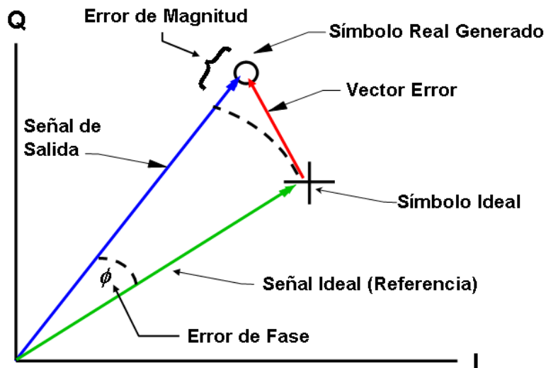
Figura 12. Magnitud del Vector Error (EVM).
