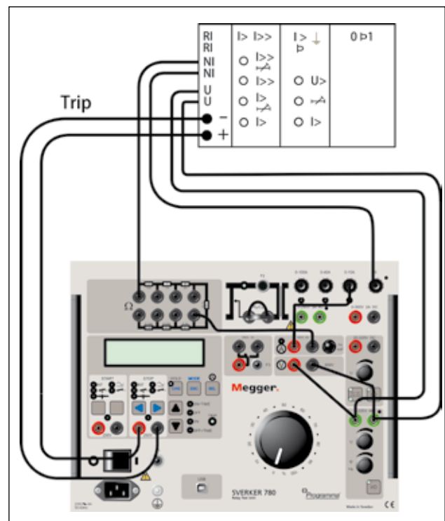
Probando el enganche y desenganche usando SVERKER 780
