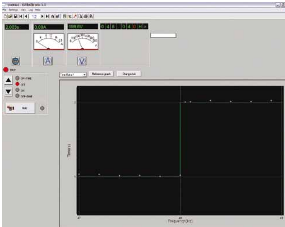
Probando relé de frecuencia con SVERKER 780
