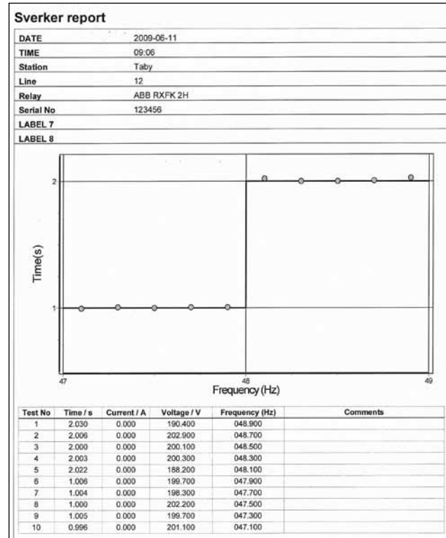
Reporte de prueba de relé de frecuencia
