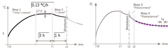
Heat Rise
