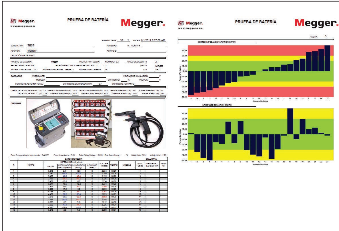
Figura 3. Preparación de informes con el PowerDB
