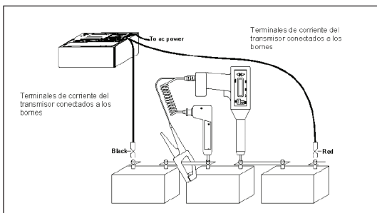
Figura 2. Configuración común de prueba
